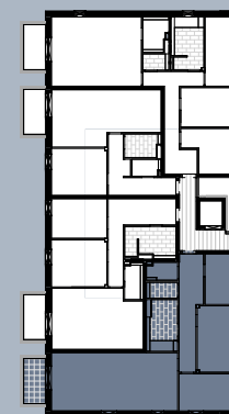
Grundriss (ohne Maßstab)
