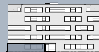
Ansicht Ost ( ohne Maßstab)
