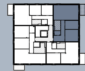
Grundriss (ohne Maßstab)
