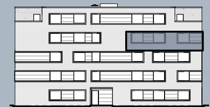
Ansicht Ost ( ohne Maßstab)
