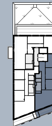
Grundriss (ohne Maßstab)
